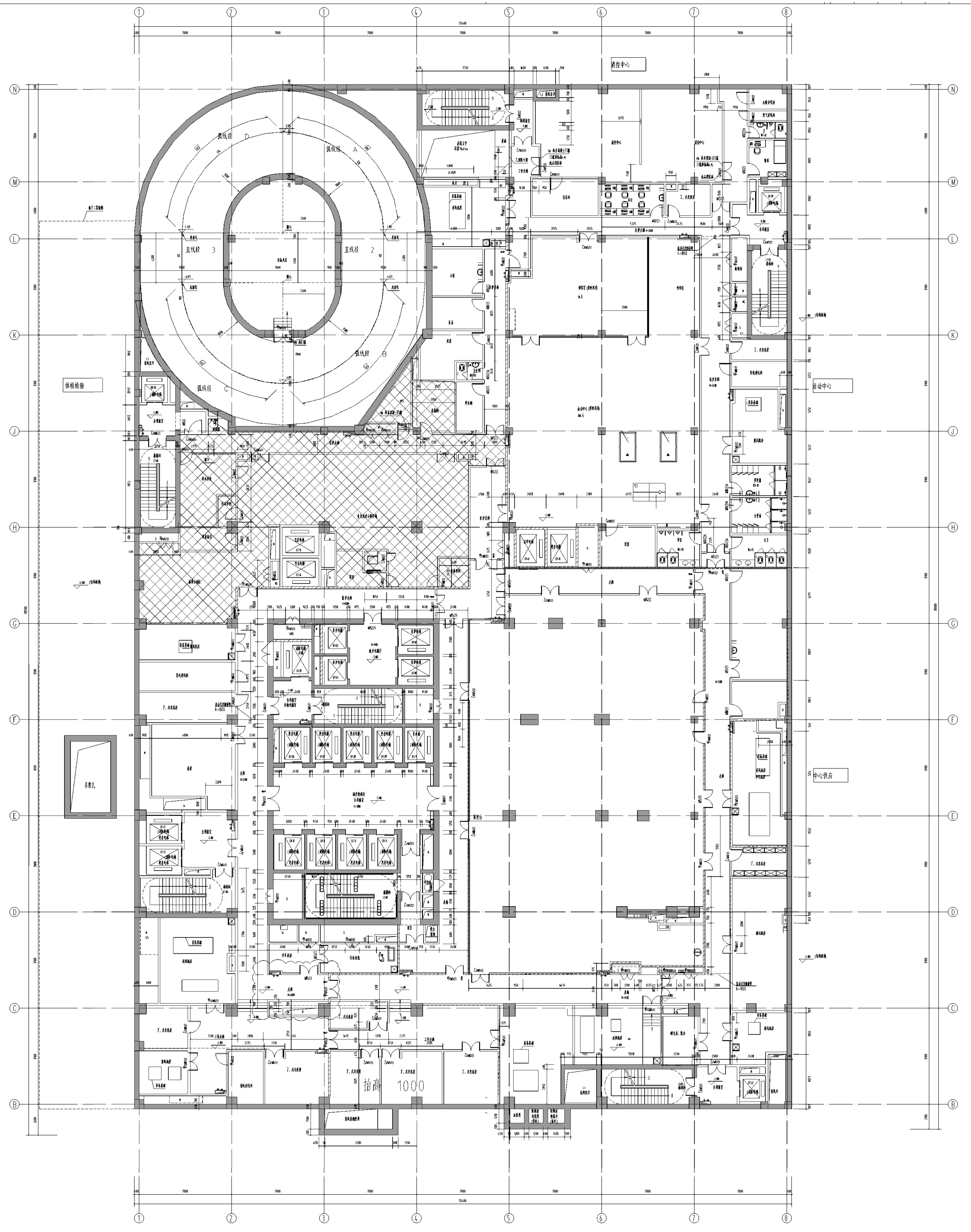
地下一层平面图 1:80 本层建筑面积:4620.97m 2
